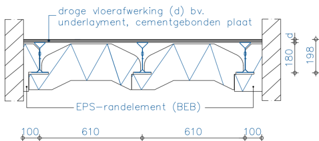
liggers h.o.h. 610
