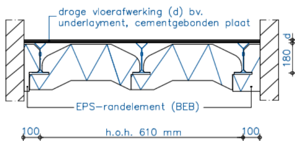
Doorsnede PS-renovatievloer Droog
