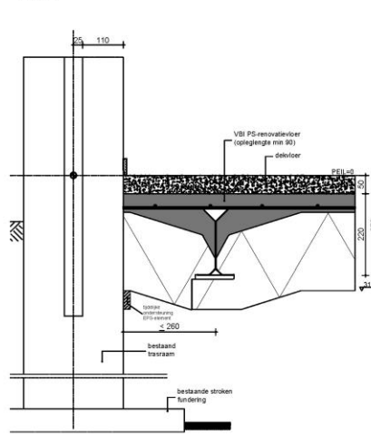
Begane grondvloer - langsgewel IIa-2
