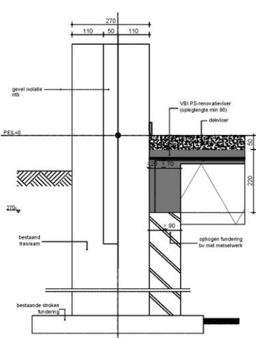
Begane grondvloer - kopgevel Ia-2
