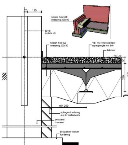
Begane grondvloer - langsgewel IIa-1
