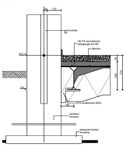
Begane grondvloer - langsgewel IIa-3
