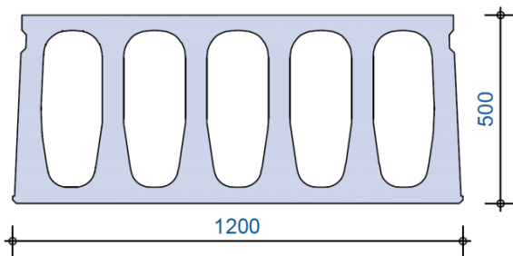
Doorsnede
