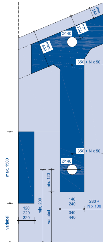
Mogelijkheden voor (fabrieksmatige) leidingsleuven
