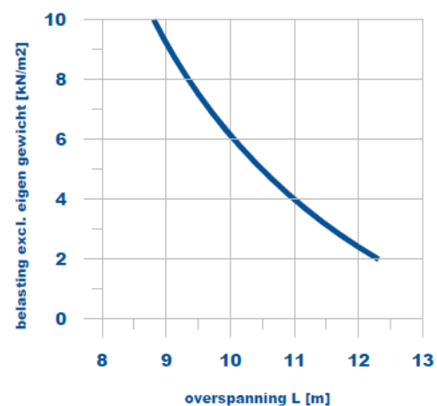
Draagvermogen grafiek
