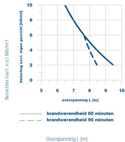
Draagvermogen grafiek
