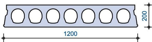
Doorsnede
