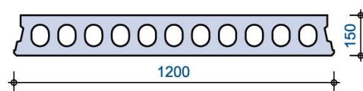
Doorsnede
