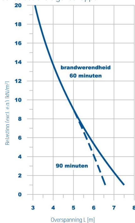
Draagvermogen grafiek
