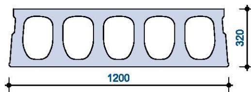
Doorsnede
