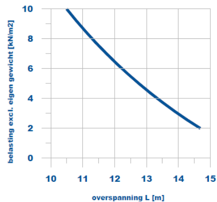
Draagvermogen grafiek
