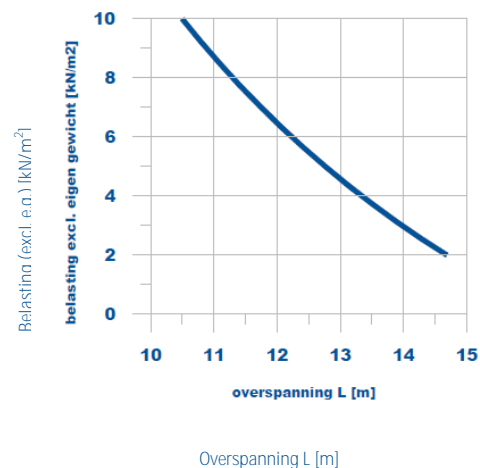
Draagvermogen grafiek
