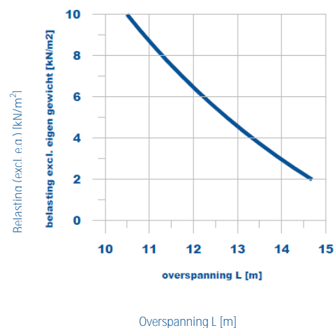
Draagvermogen grafiek
