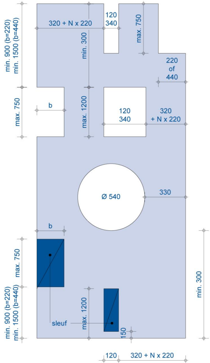
Mogelijkheden voor het fabrieksmatig aanbrengen van sparingsen
