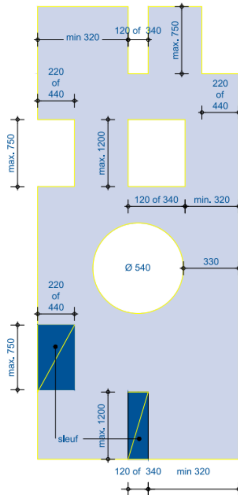
Mogelijkheden voor het fabrieksmatig aanbrengen van sparingsen
