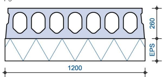
Doorsnede
