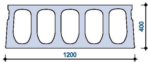
Doorsnede
