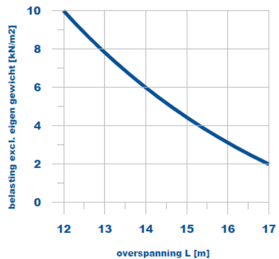
Draagvermogen grafiek
