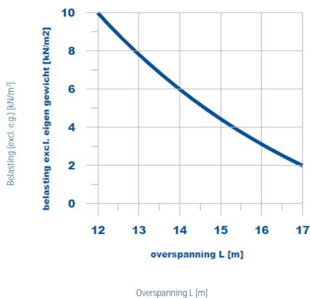
Draagvermogen grafiek
