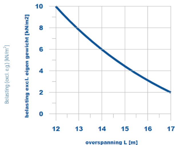
Draagvermogen grafiek
