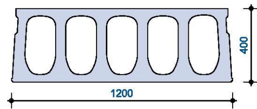
Doorsnede
