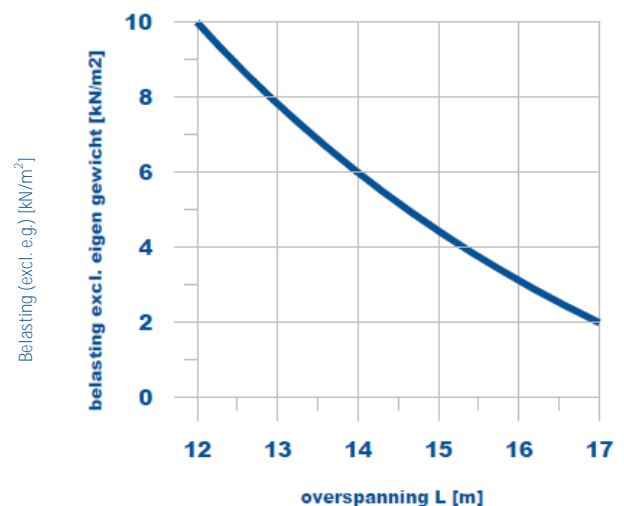
Draagvermogen grafiek
