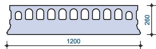
Doorsnede
