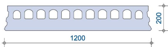
Doorsnede
