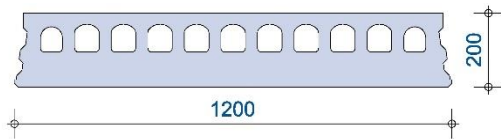
Doorsnede
