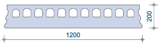
Doorsnede
