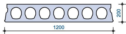
Doorsnede
