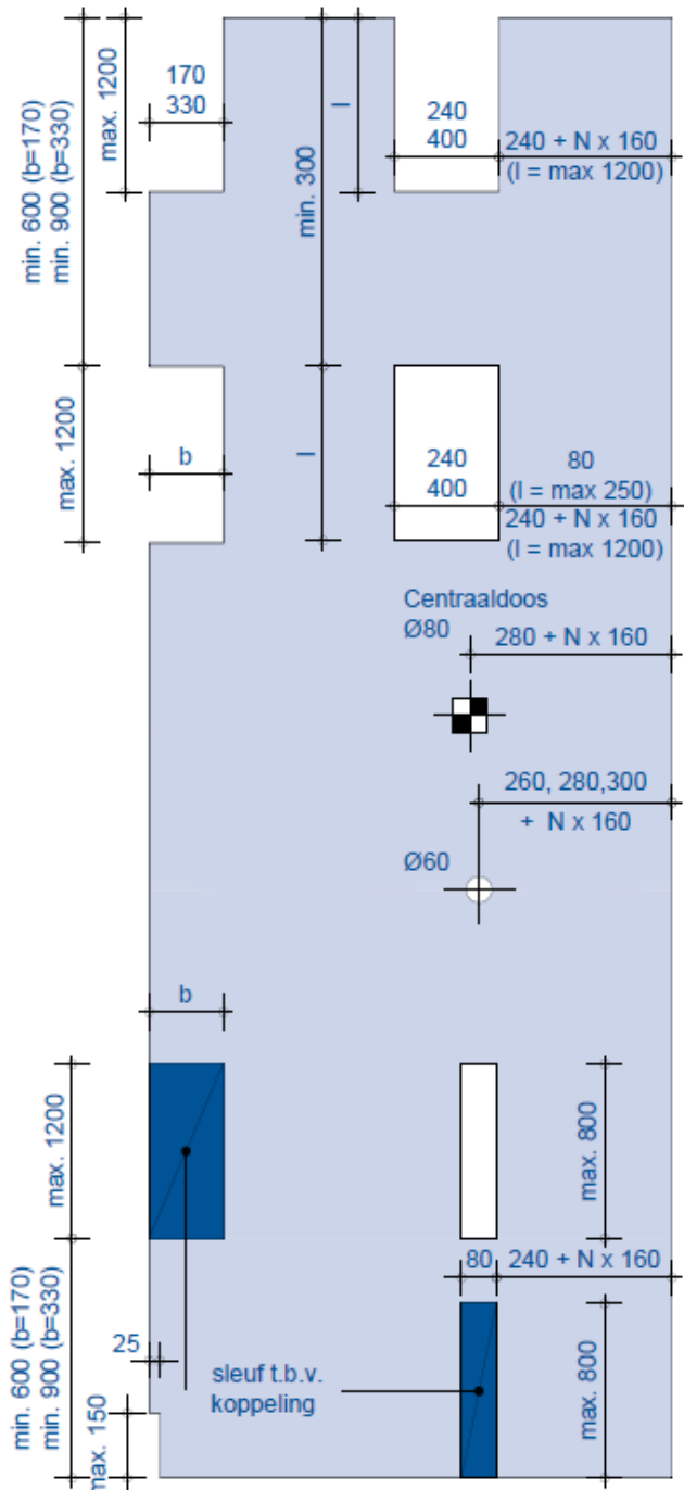
Mogelijkheden voor het fabrieksmatig aanbrengen van sparingen
