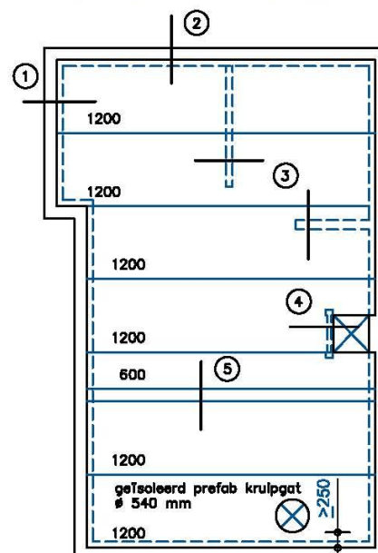
LEGPLAN en DETAIL AANDUIDINGEN
