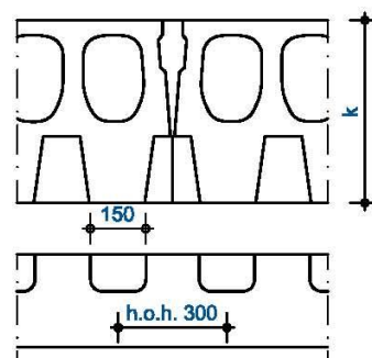
AANZICHTEN RANDOPLEGGING
