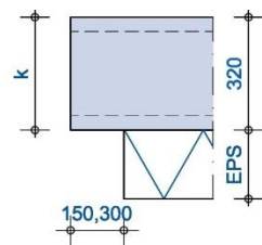
Ongeïsoleerde oplegging
