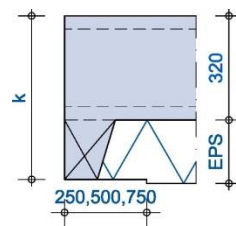
Geïsoleerde oplegging
