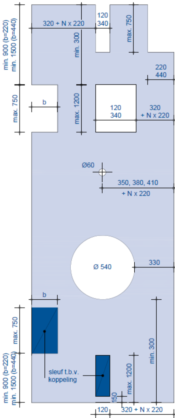
Mogelijkheden voor het fabrieksmatig aanbrengen van sparingen
