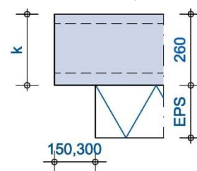
Ongeïsoleerde oplegging
