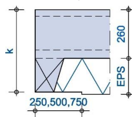
Geïsoleerde oplegging
