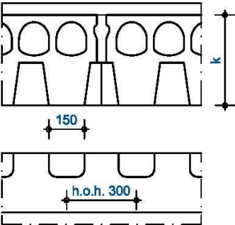
AANZICHTEN RANDOPLEGGING
