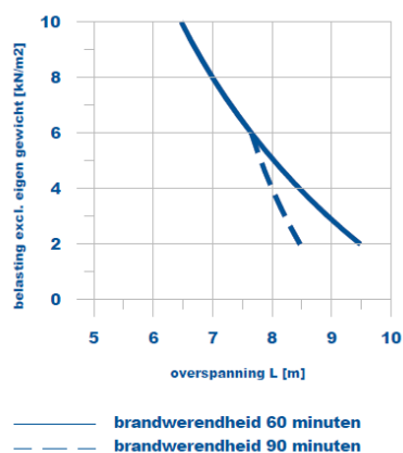
Draagvermogen grafiek
